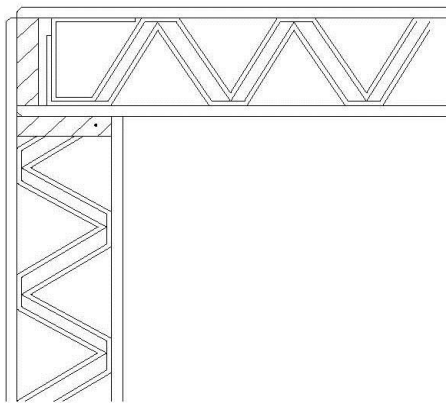
11. BIA hoekoplossing met montageplaten
