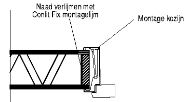
10. BIA detail montagekozijn
