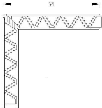
12. BIA hoekoplossing met MDF hoeklat
